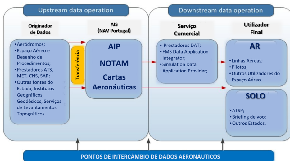
Figura 1: Representação da Cadeia de Dados Aeronáuticos “Aeronautical Data Chain” e os seus constituintes. 1
